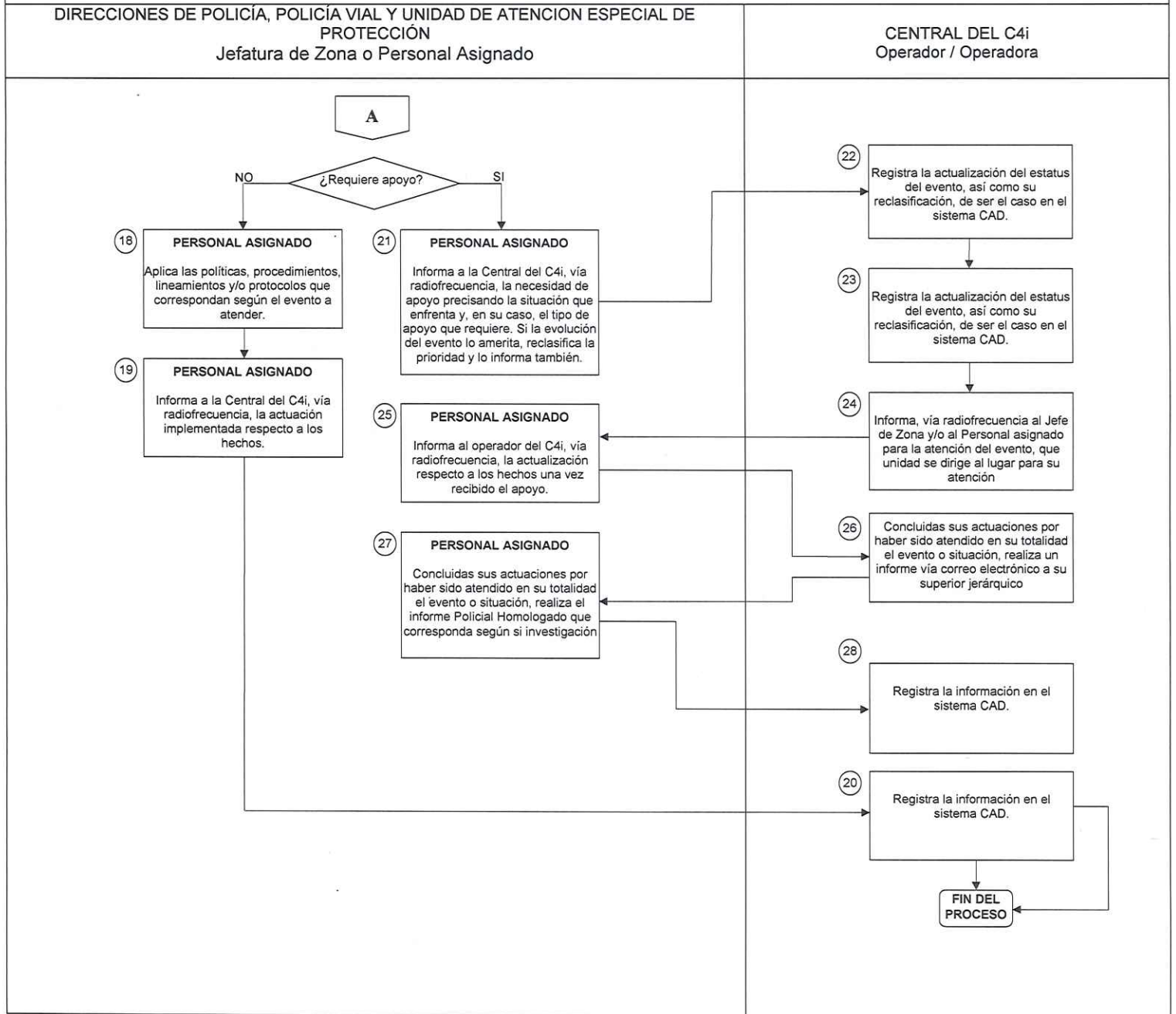
DIAGRAMA DE FLUJO DEL PROCESO RECEPCIÓN Y TRATAMIENTO DE LLAMADAS EN EL C4i SAN PEDRO HOJA #2
